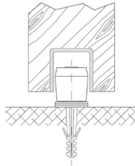
FÜHRUNGSROLLE AUS NYLON ODER MESSING MIT DÜBEL (.N58 oder .M58)
