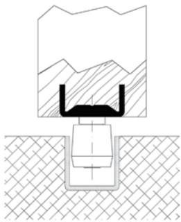
FÜHRUNGSROLLE AUF FLANSCH AUS NYLON ODER MESSING (.N00 oder .M00)
