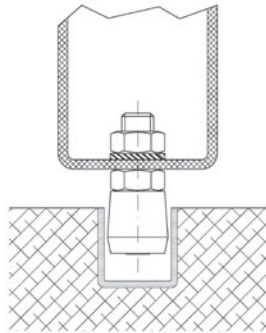
FÜHRUNGSROLLE MIT SCHRAUBVERBINDUNG AUS NYLON ODER MESSING (.N49 oder.M49)
