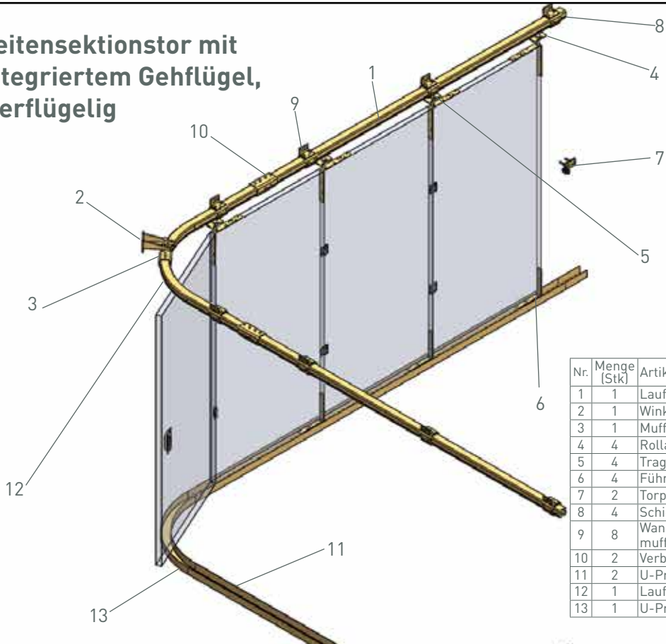
Seitensektionstor zur Automatisierung
