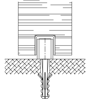
GLEITSTÜCK MIT DÜBEL UND SENK KOPFSCHAUBEN (.U54)
